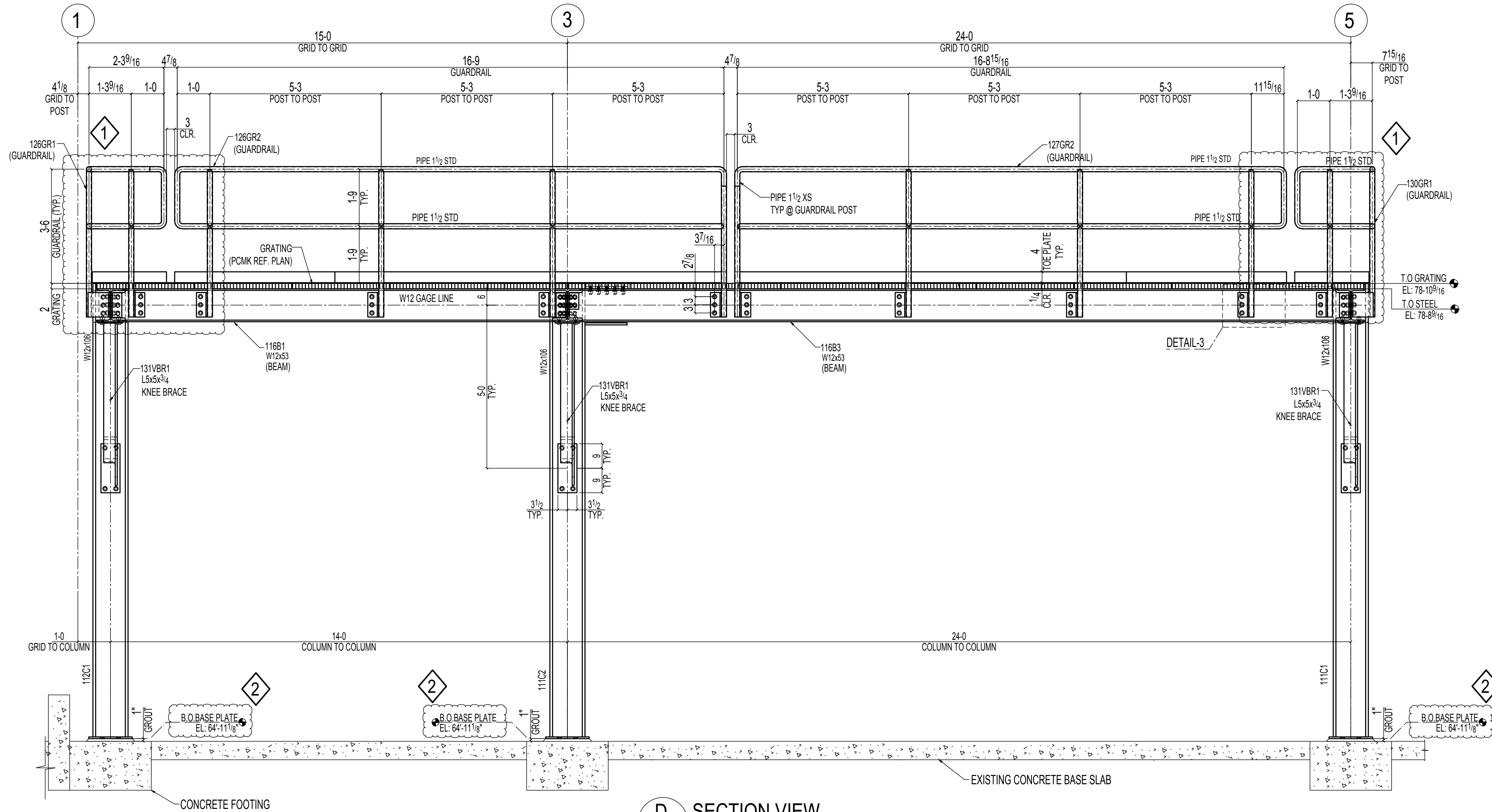
D SECTION VIEW E107
