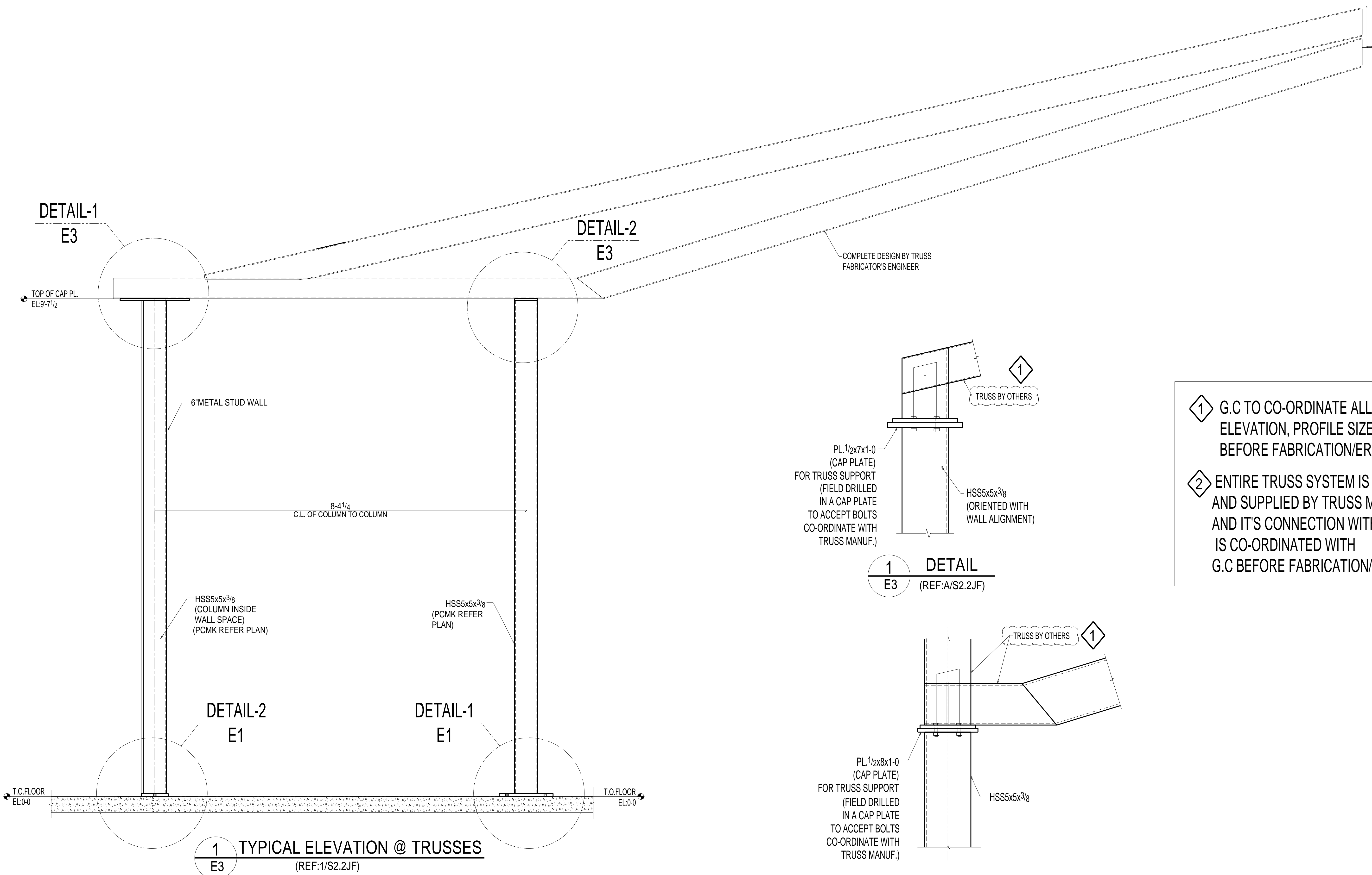
2 DETAIL E3 (REF:B/S2.2JF)
