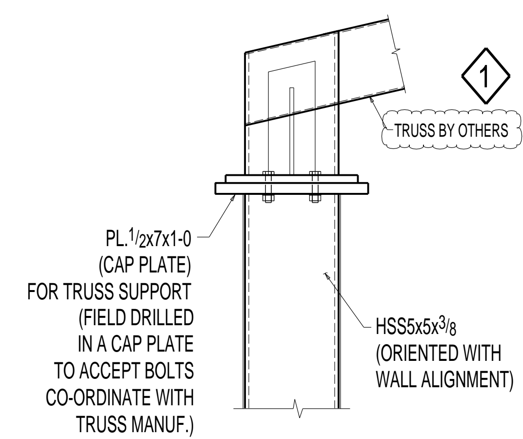
1 DETAIL E3 (REF:A/S2.2JF)
