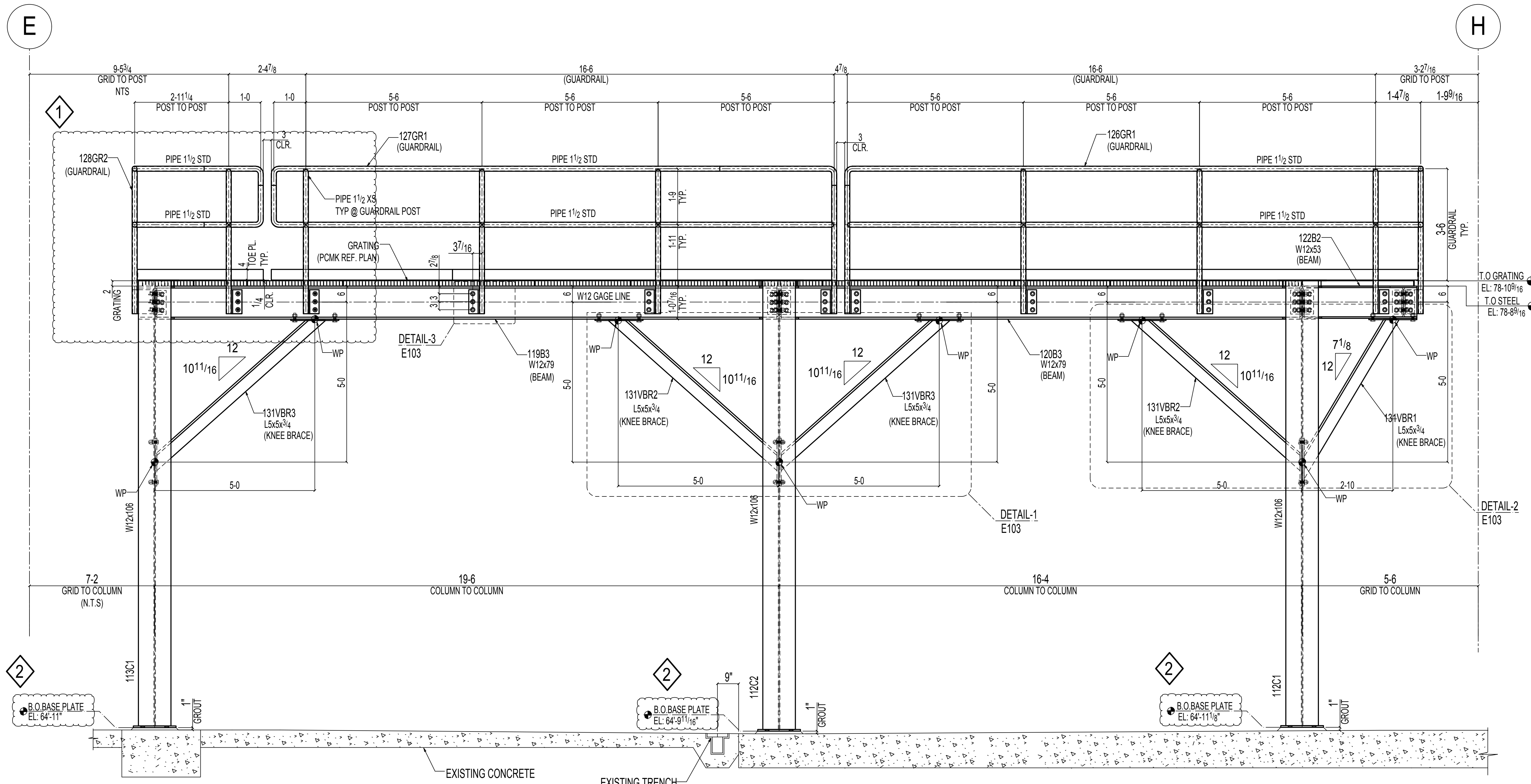
A SECTION VIEW E104
